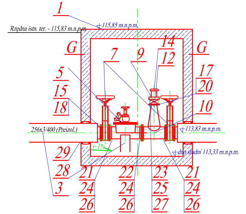
Przekrój D - D
