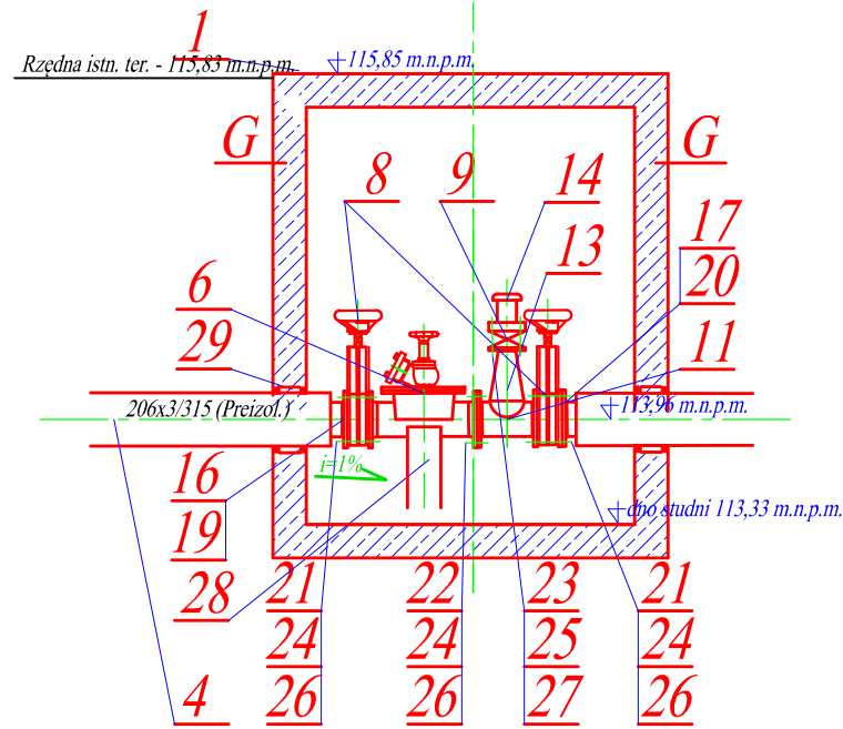
Przekrój C - C
