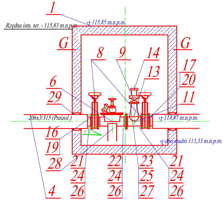
Przekrój E - E
